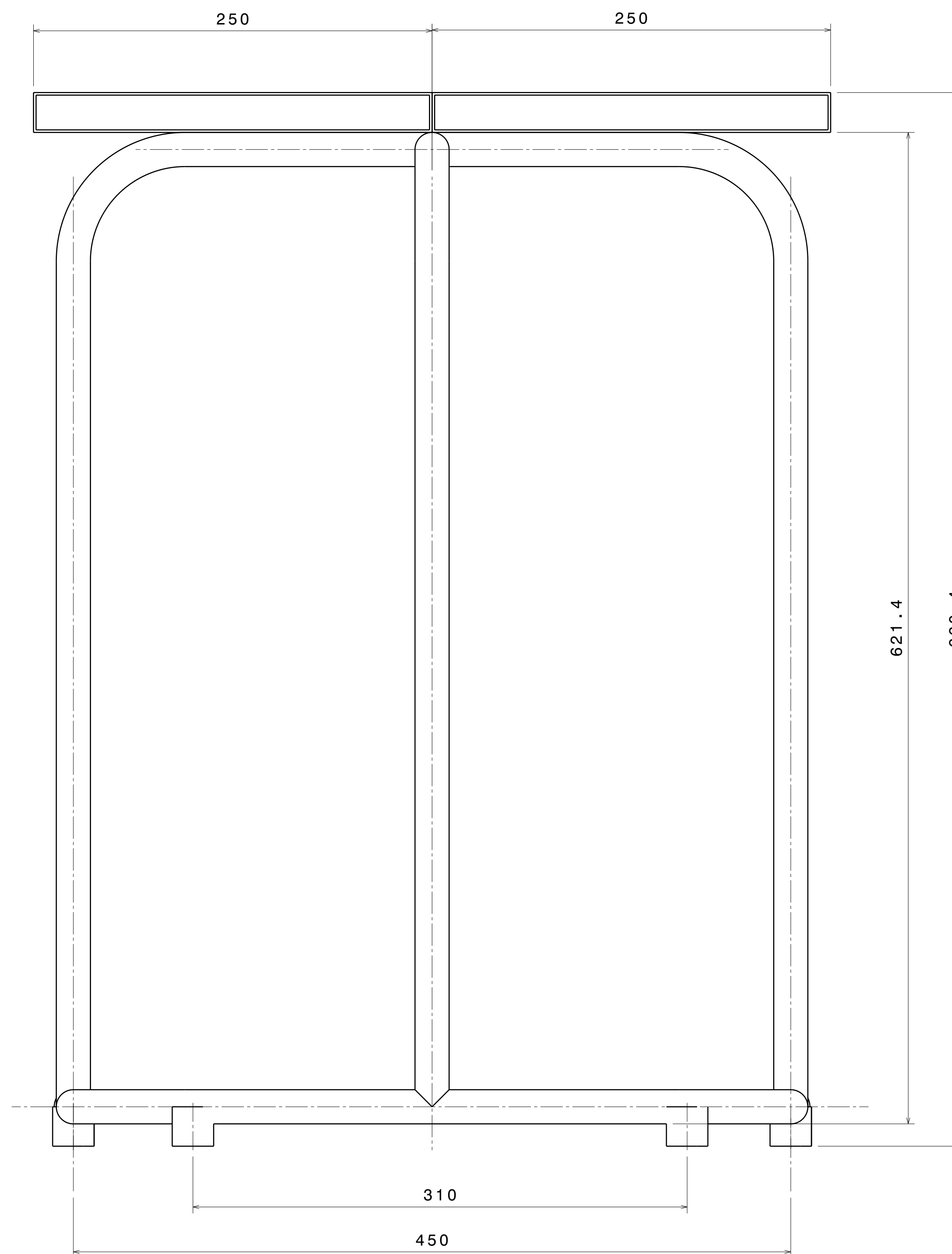
Right view Scale: 1:2
