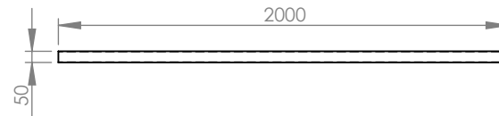
ITEM 7 SHS 50X50X2.0X2000
