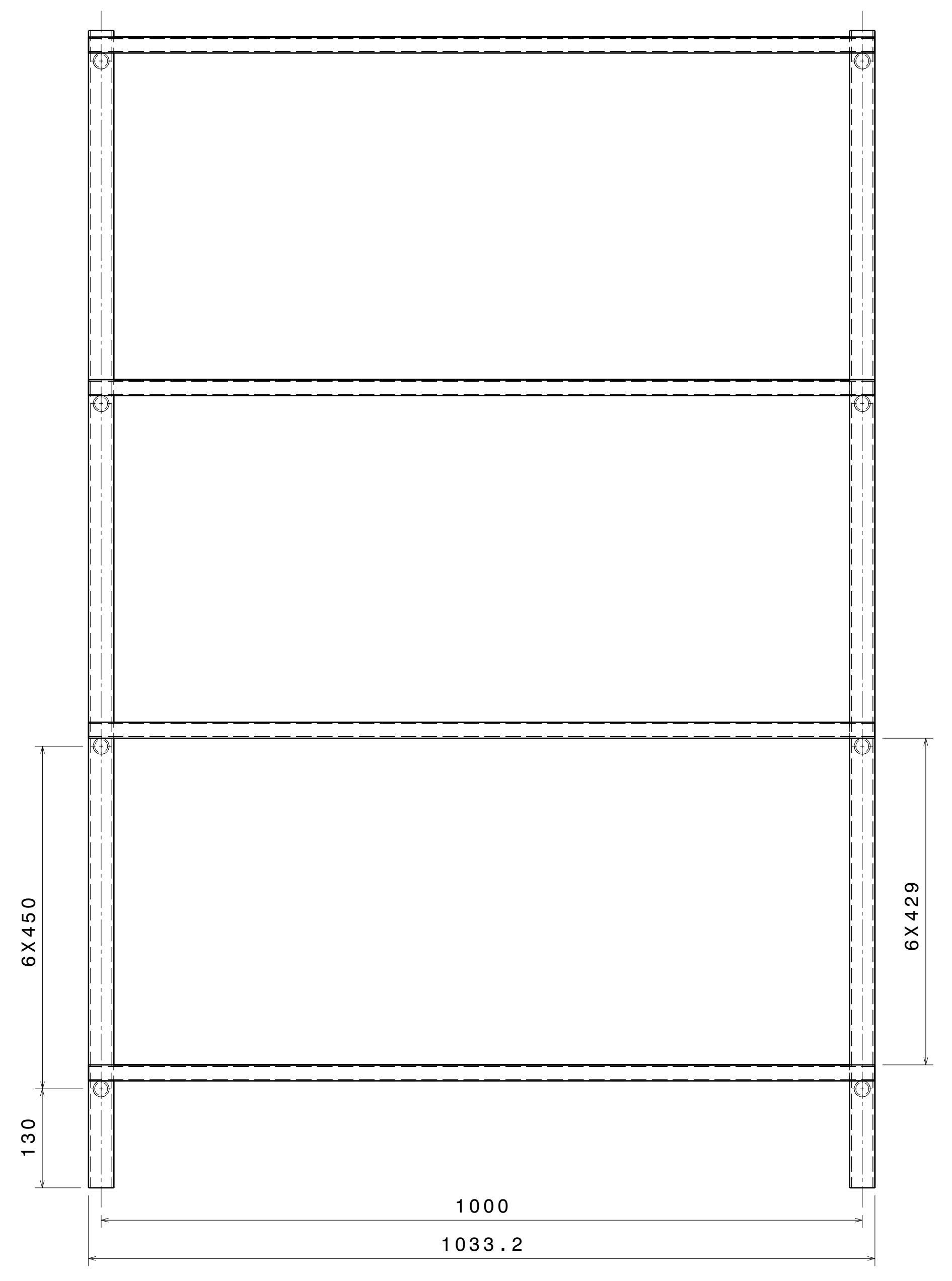
Front view Scale: 1:5
