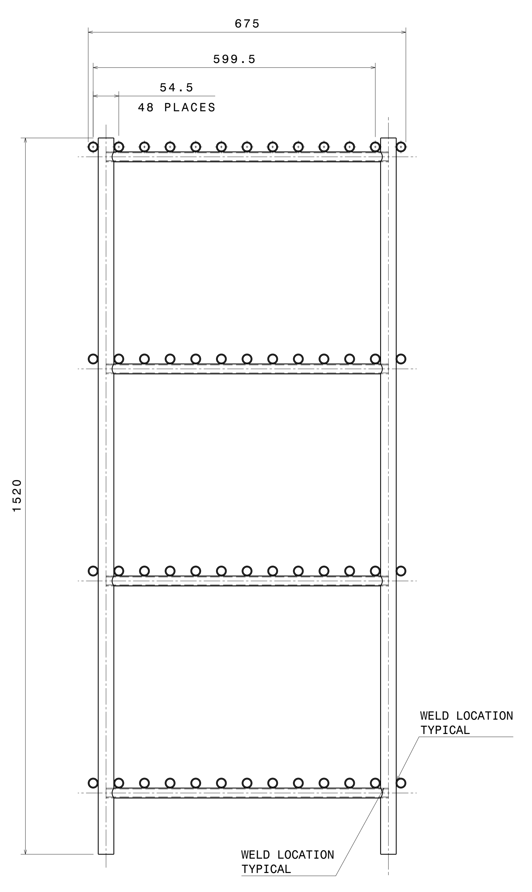
Right view Scale: 1:5
