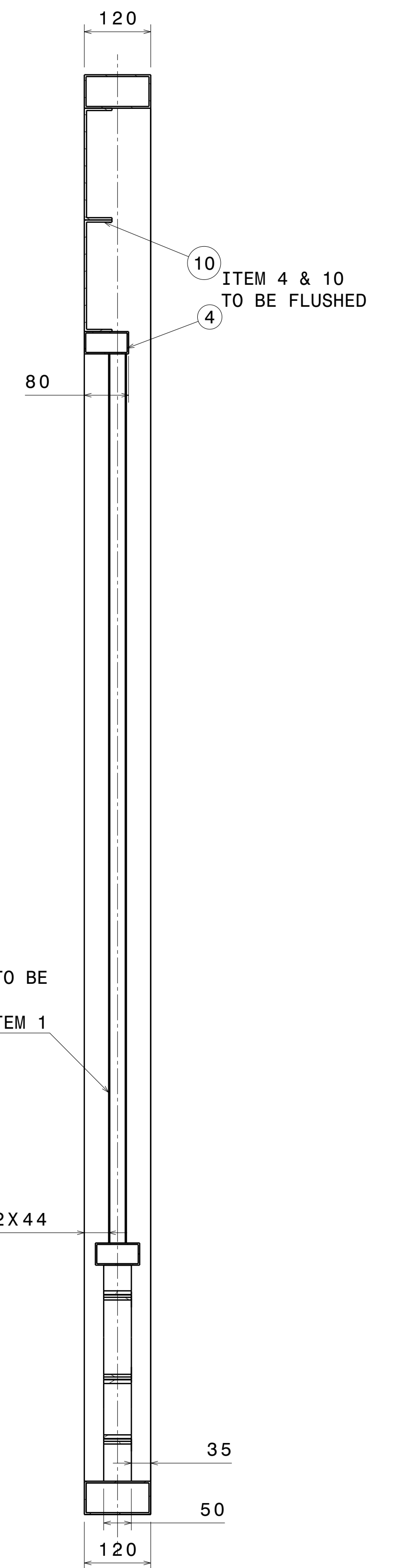
Section view A-A Scale: 3:20
