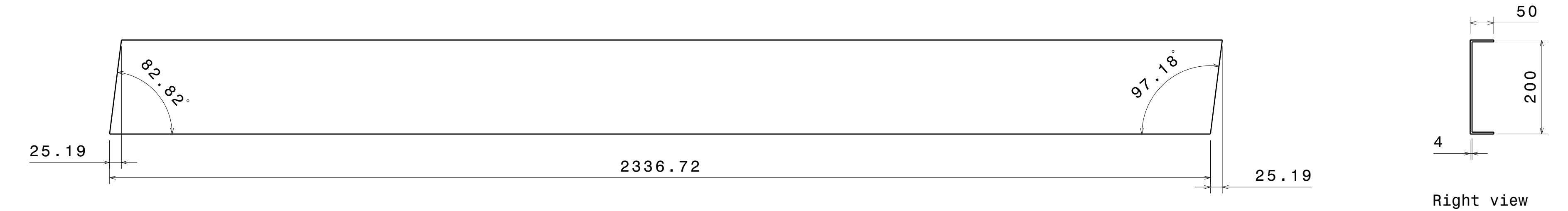
ITEM 9, QTY 2 LEFT SIDE
