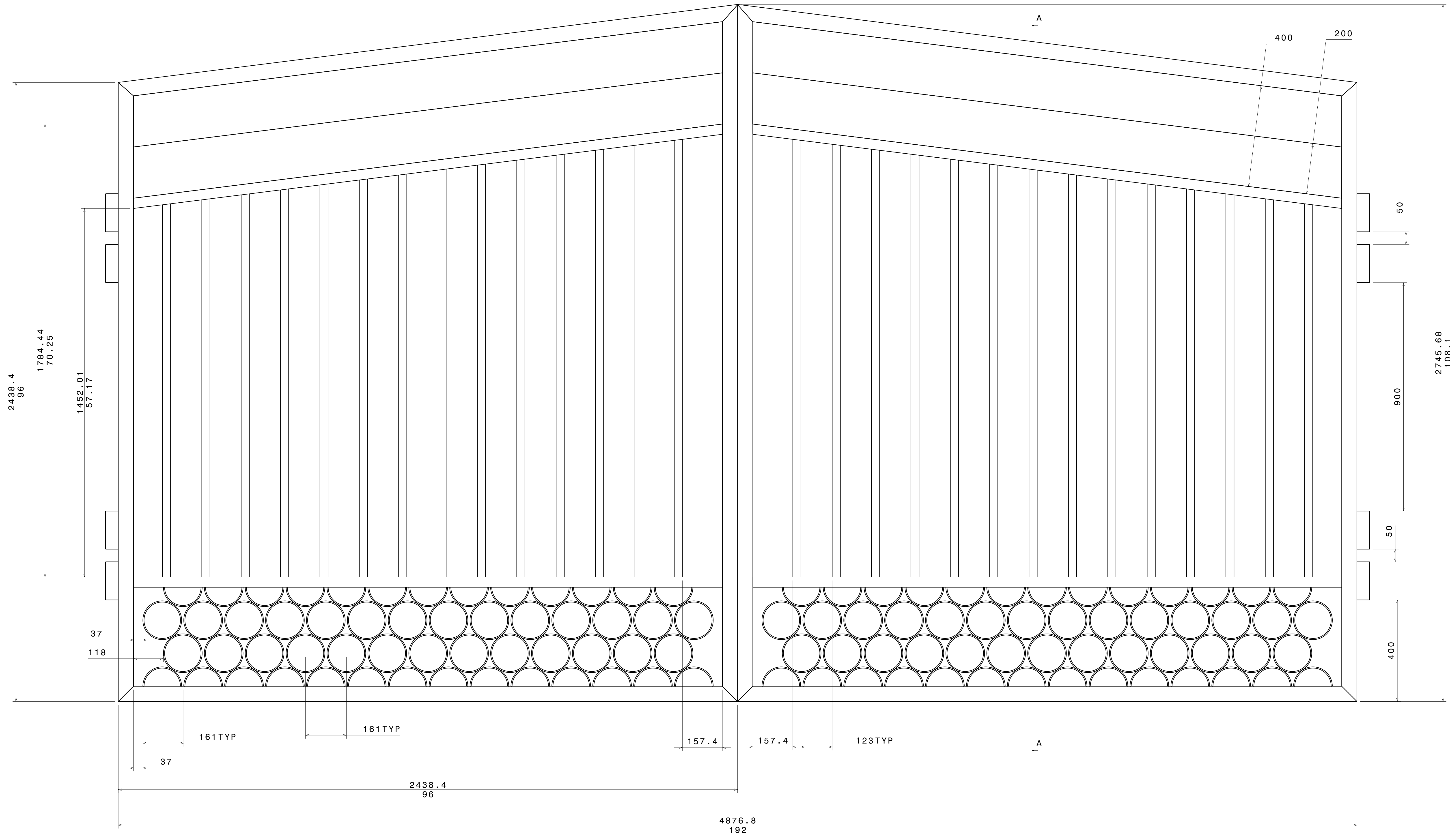
Front view Scale: 3:20
