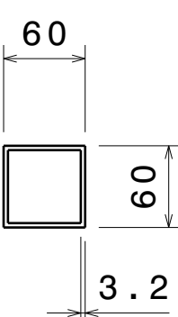
Right view Scale: 1:5
